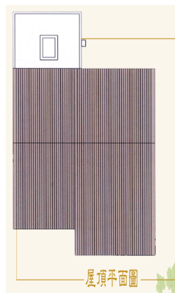
〔圖 2〕屋頂平面圖
